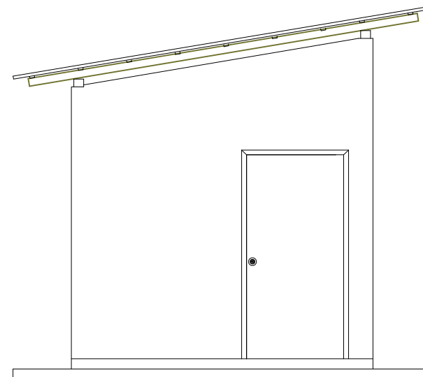
Fachada ESCALA: 1/50
