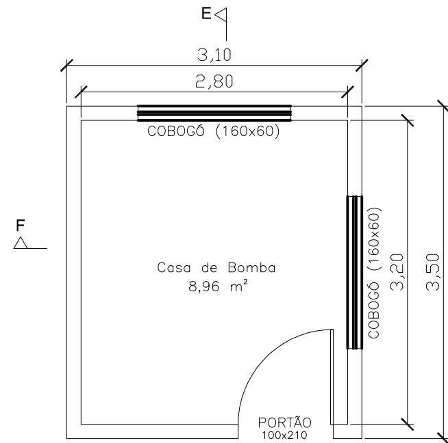
Planta Baixa ESCALA: 1/50
