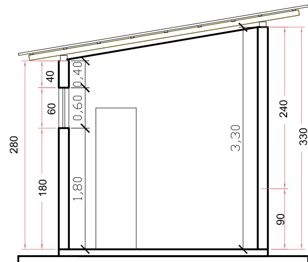
Corte FF ESCALA: 1/50
