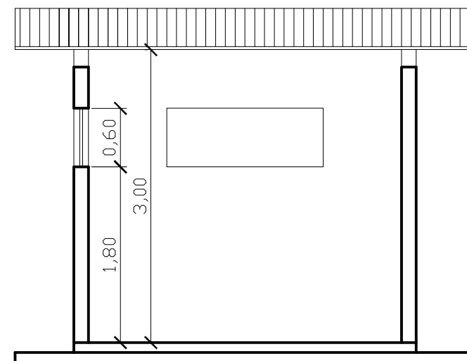
Corte EE ESCALA: 1/50
